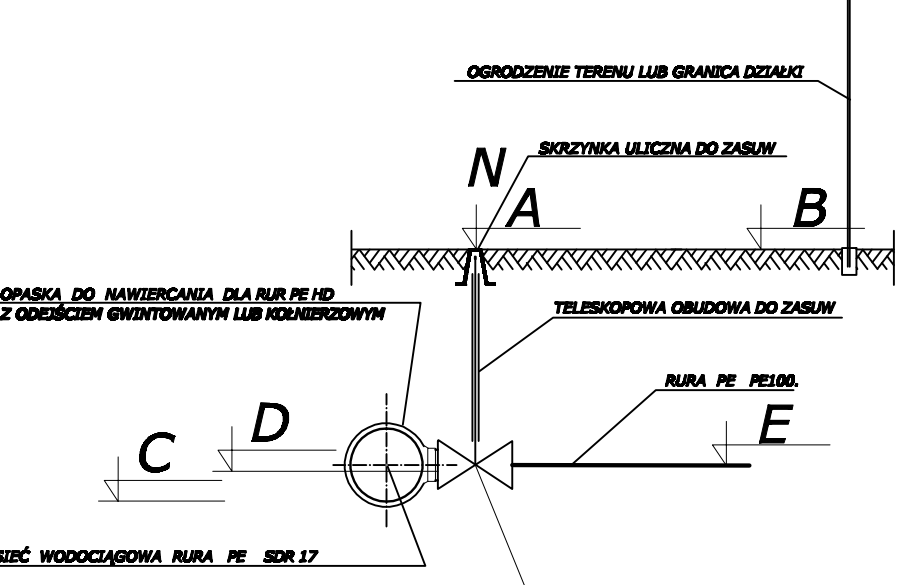
PROFIL PRZYŁĄCZA POŁĄCZONEGO Z ISTNIEJĄCYM RUROCIĄGIEM
